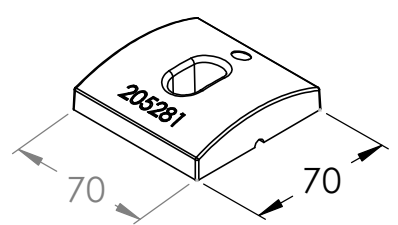
DÉTAILS DES CALES CYLINDRIQUE
