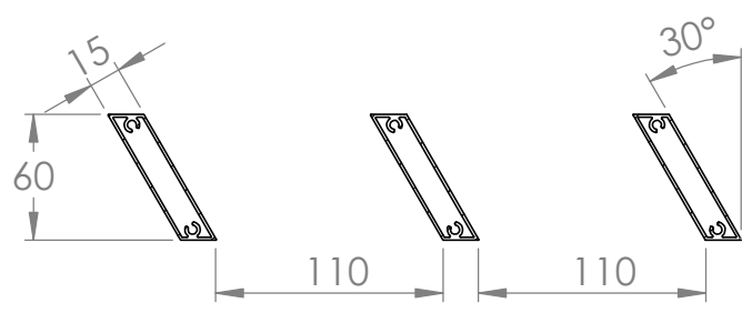
PROFIL BARREAUDAGE
