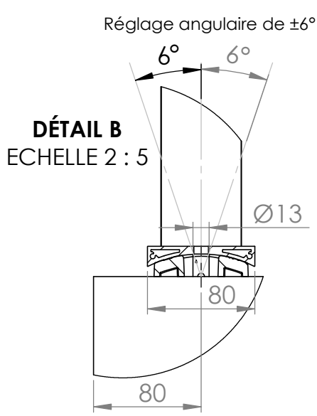
PROFIL BARREAUDAGE
